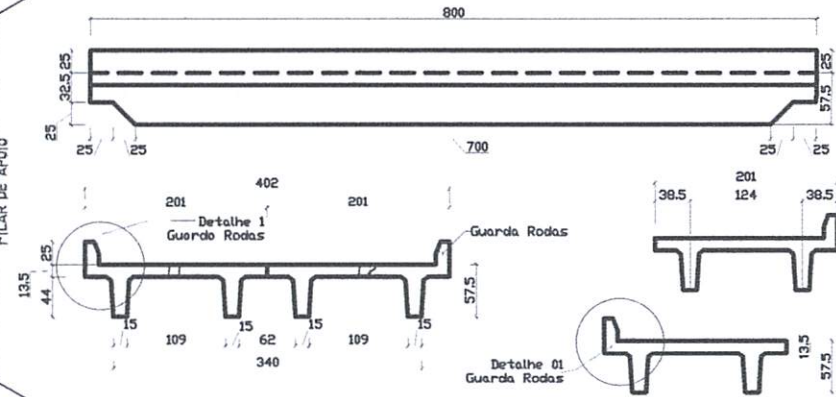
4 DETALHAMENTO (LI/L2) Esc. 1:100
