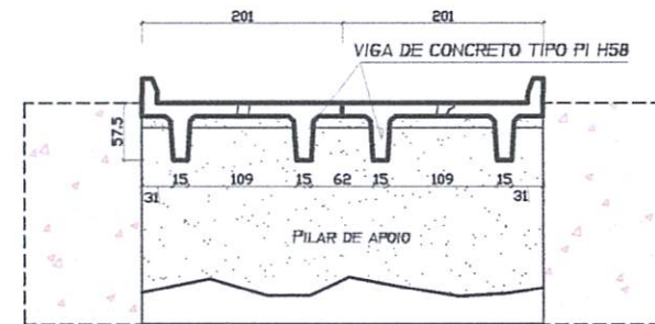
3 CORTE A'A Esc. 1:100
