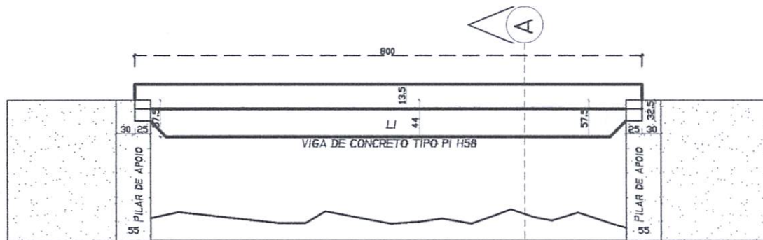
2 VISTA LATERAL Esc. 1:100
