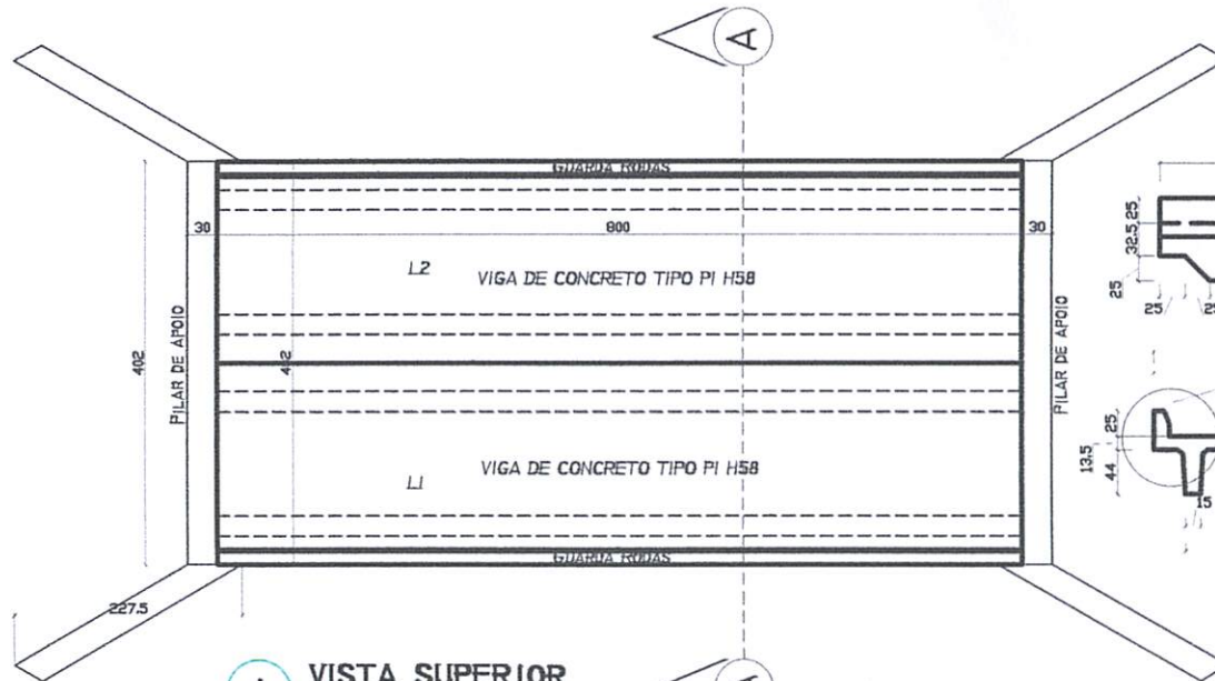
1 VISTA SUPERIOR Esc. 1:100
