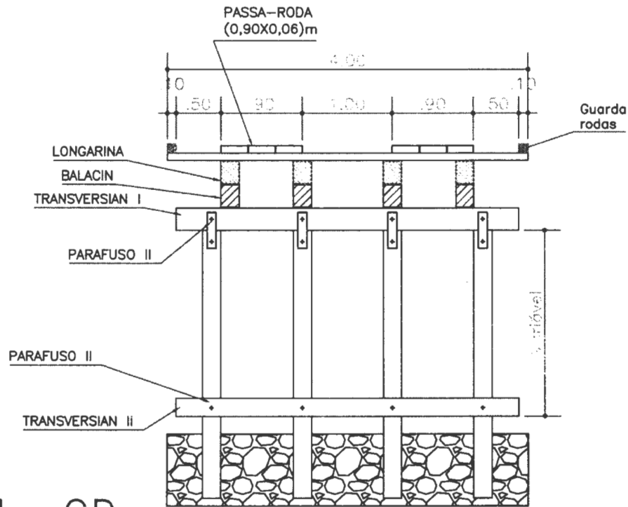
Corte CD
